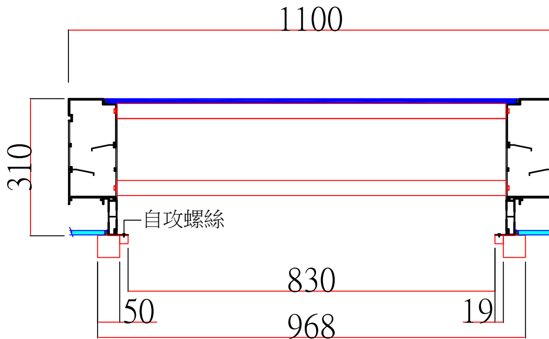
不銹鋼方管採光罩安裝剖面圖
