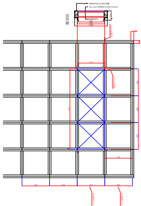
三樑續接
