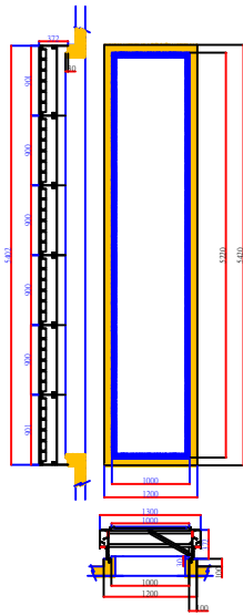
RC-續接6樁施工圖
