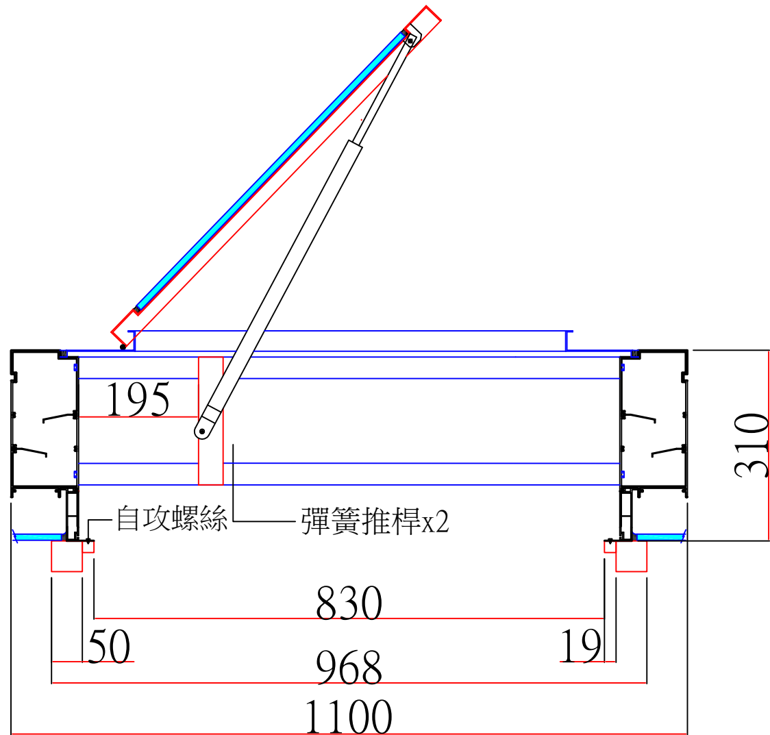
不銹鋼方管採光罩安裝剖面圖
