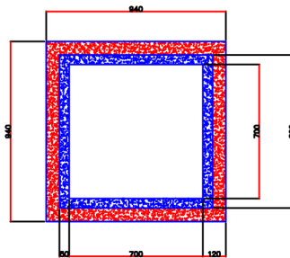
RC-最佳單組施工圖
