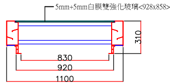
剖面圖
