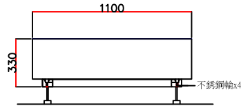
右側立面
