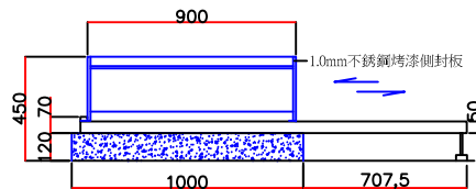
正立面
