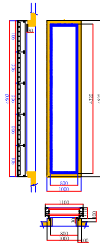
RC-續接5樁施工圖
