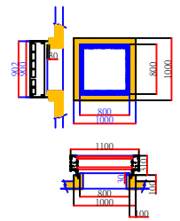
RC-續接1樁施工圖
