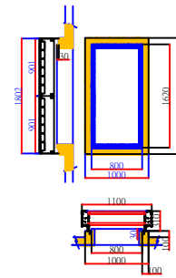
RC-續接2樁施工圖
