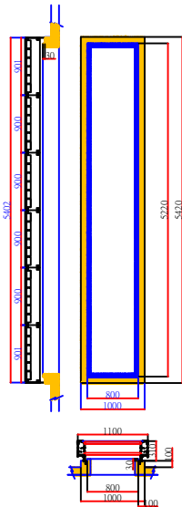
RC-續接6樁施工圖
