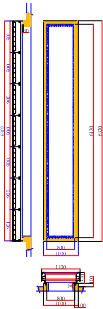
RC-續接7樁施工圖
