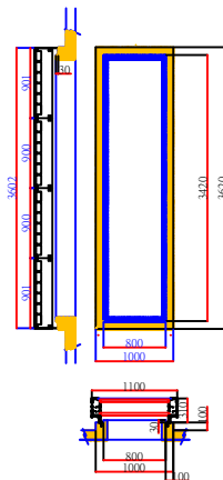
RC-續接4樁施工圖
