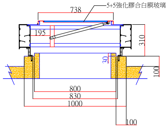
RC-1樁施工圖 RC座孔徑示意圖(泥作完成面)
