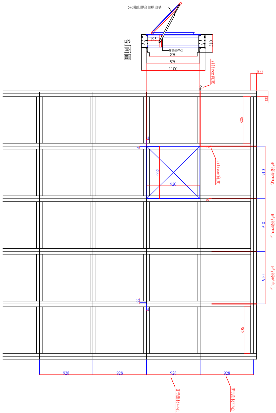
H型鋁料採光罩-孔洞尺寸圖
